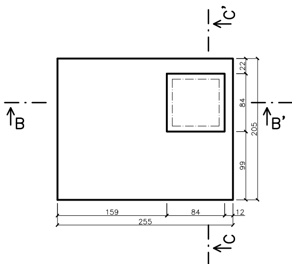
PUDORYS
