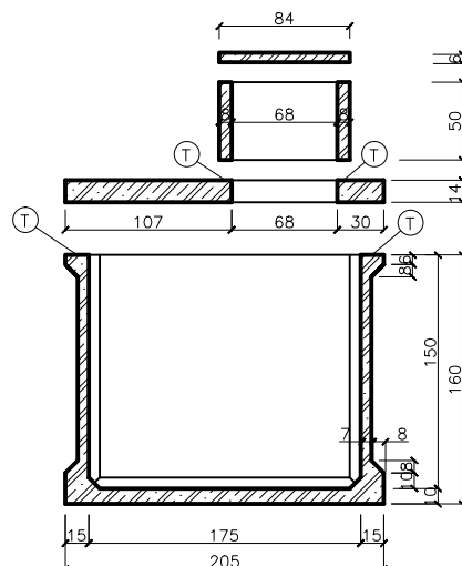
ŘEZ C–C'
