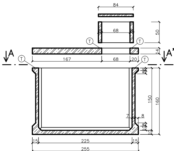
ŘEZ B–B'
