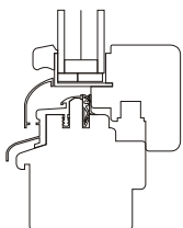
VARIANTA PRO ZASKLENÍ O SÍLE 28mm (NAPŘ. HEAT MIRROR- U sklo = 0,7W/m 2 K)
