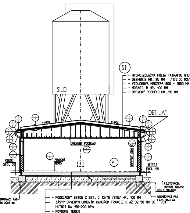
rez 07 sklad soli
