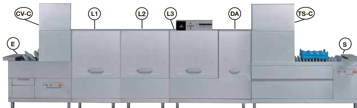
Skladba modulů a doplňků FI-6000 I s kondenzátorem par CV-C a sušicím tunelem TS-C
