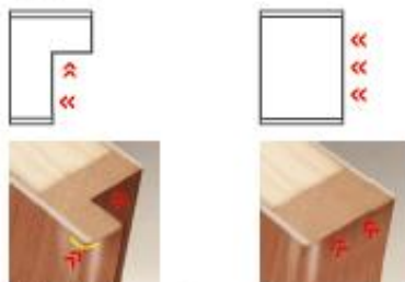
faľcová hrana dverí - s polodrážkou
