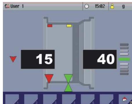
ALU S - stanovení libovolné polohy obou rovin
