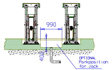
Cut A-A
