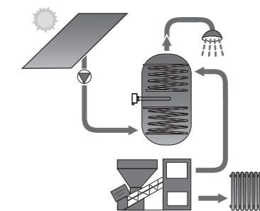
Obr 4 systém s kotlem na biomasu doplněným elektrickým tělesem
